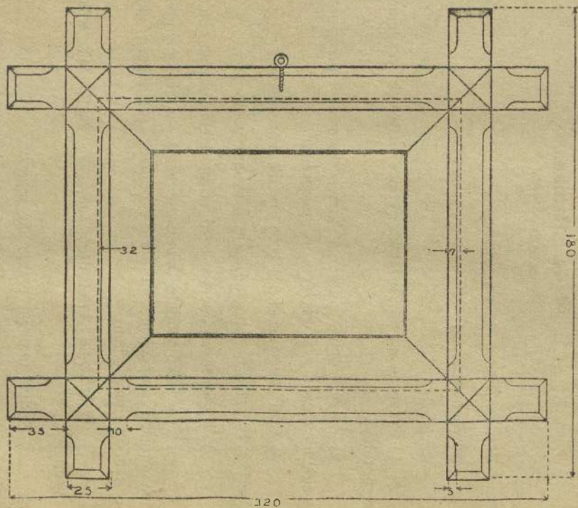
№ 44 Ramka.
