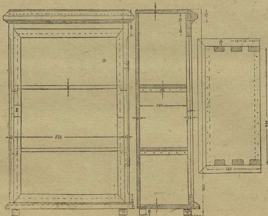
№ 61. Szafka na bibliotekę lub na roboty slöjdowne.
